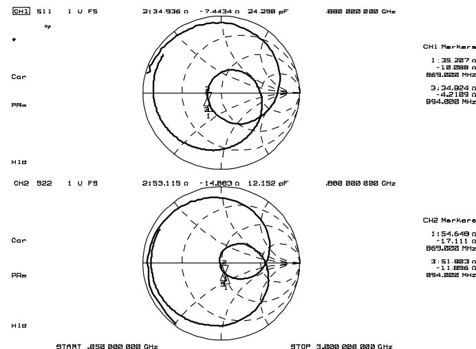
Zin, Zout
