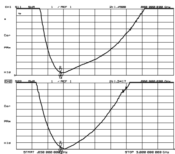
VSWR
