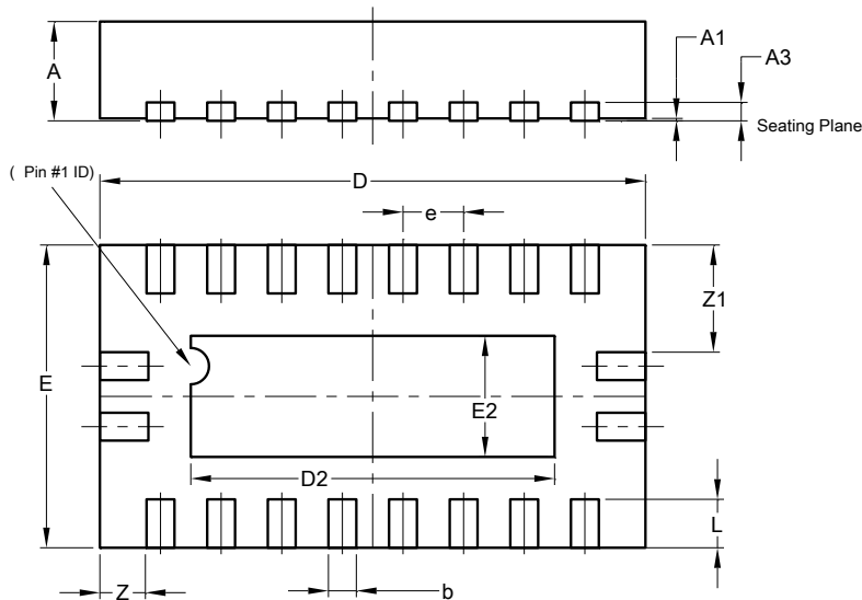
V-QFN4525-20
