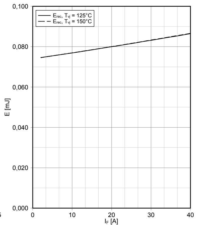
スイッチング損失 ダイオード、スリー・レベル (Typical) switching losses Diode, 3-Level (typical) E_{rec} = f(I_F) R_{Gon} = 3,9 \Omega , V_{CE} = 300 \text{ V}
