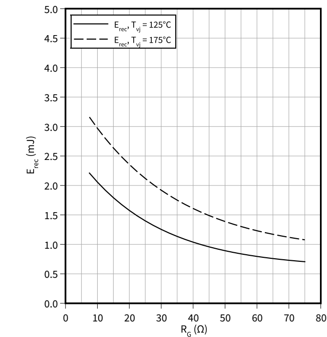
开关损耗（典型），二极管,逆变器 E_{rec} = f(R_G) I_F = 50\ \text{A} , V_R = 600\ \text{V}
