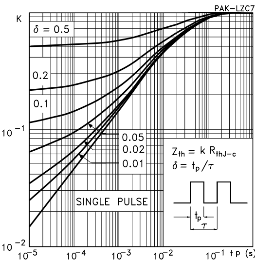
Thermal Impedance
