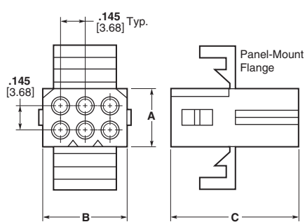
Receptacle
