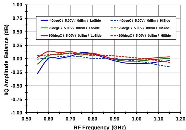
I/Q Amplitude Error vs. T CASE
