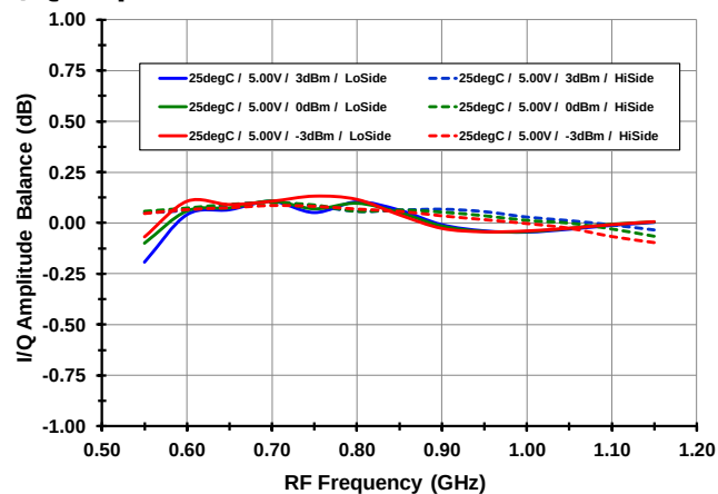
I/Q Amplitude Error vs. LO level
