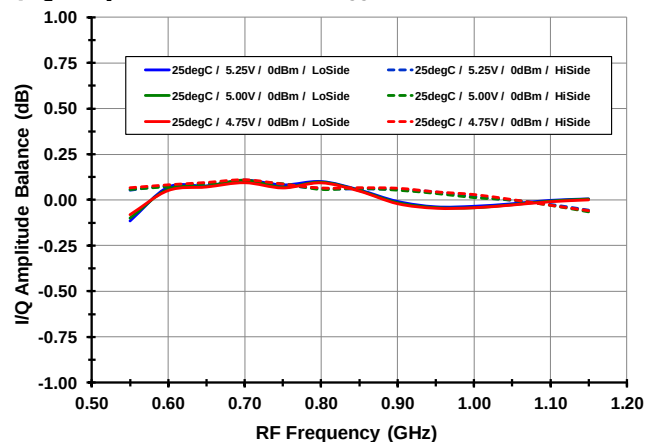
I/Q Amplitude Error vs. V CC
