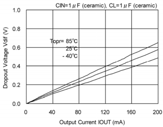
XC6219x182
