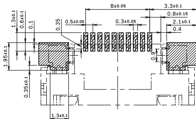
推奨取り付け寸法 (コネクタ搭載側) MOUNTING LAYOUT (CONN. MOUNTING SIDE)
